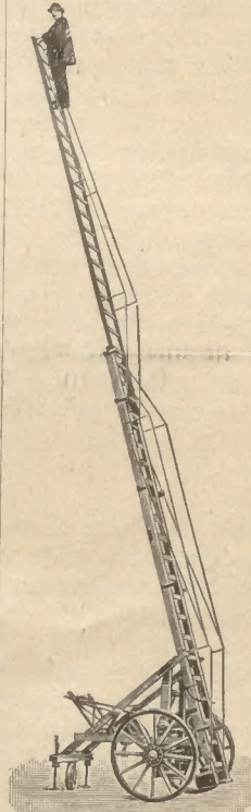
Mechanische 2-Rad-Leiter. Konstruktion B. (ohne Stützen) ganz ausgezogen 12 m hoch, 78 Grad nach vorn geneigt. In diesem Zustande von 2-3 Mann bestieigbar.
